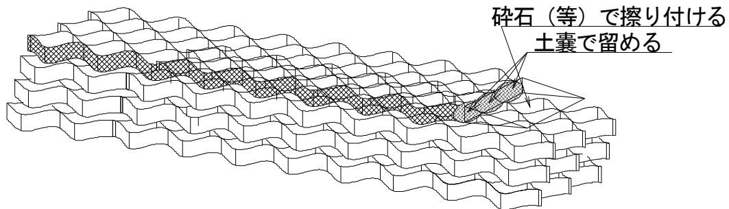
天端段差部処理図
